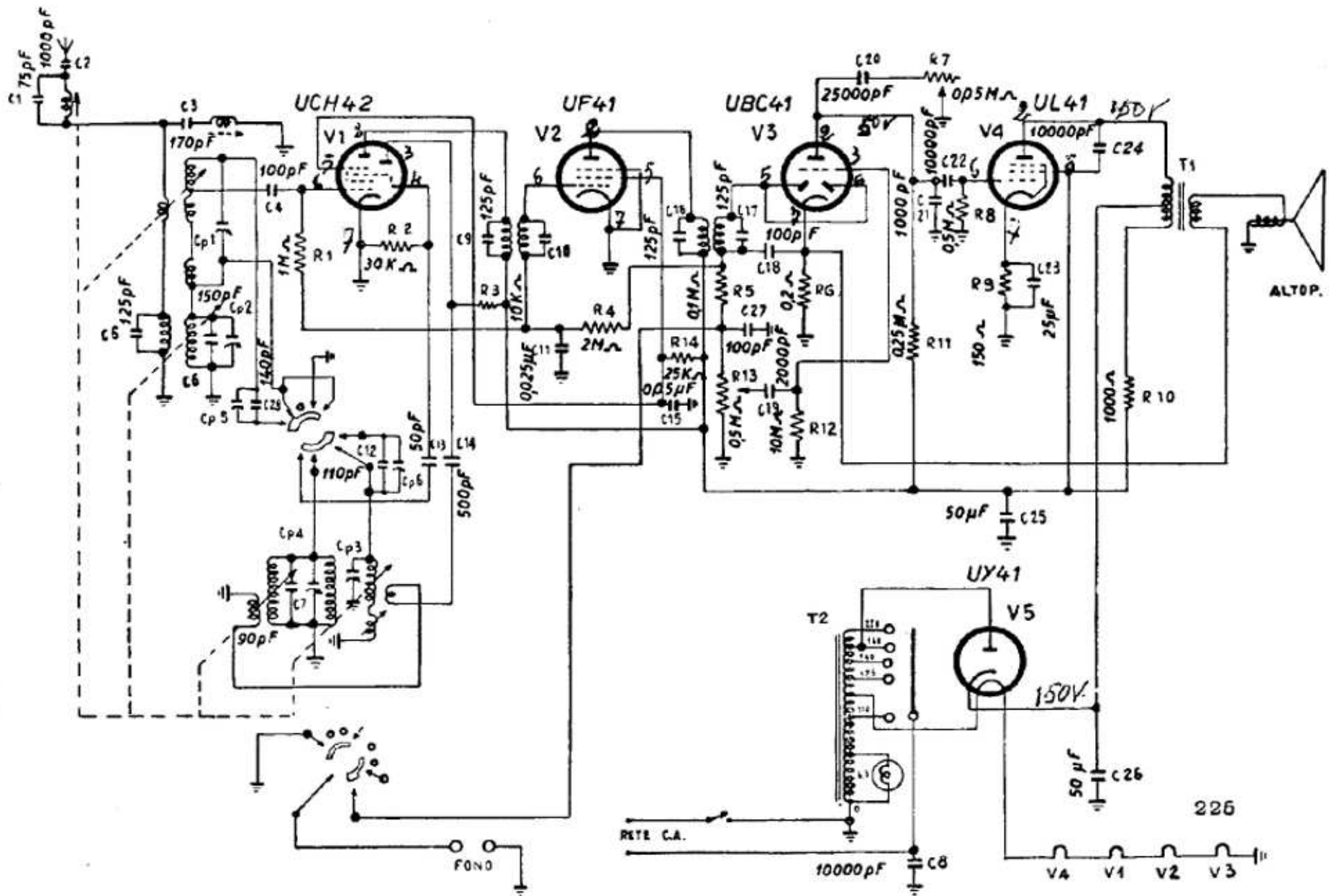
ALLOCCIO BACCHINI - Mod. 225. Ricevitore provvisto di controreazione fissa in BF. Media frequenza 465 kc.
